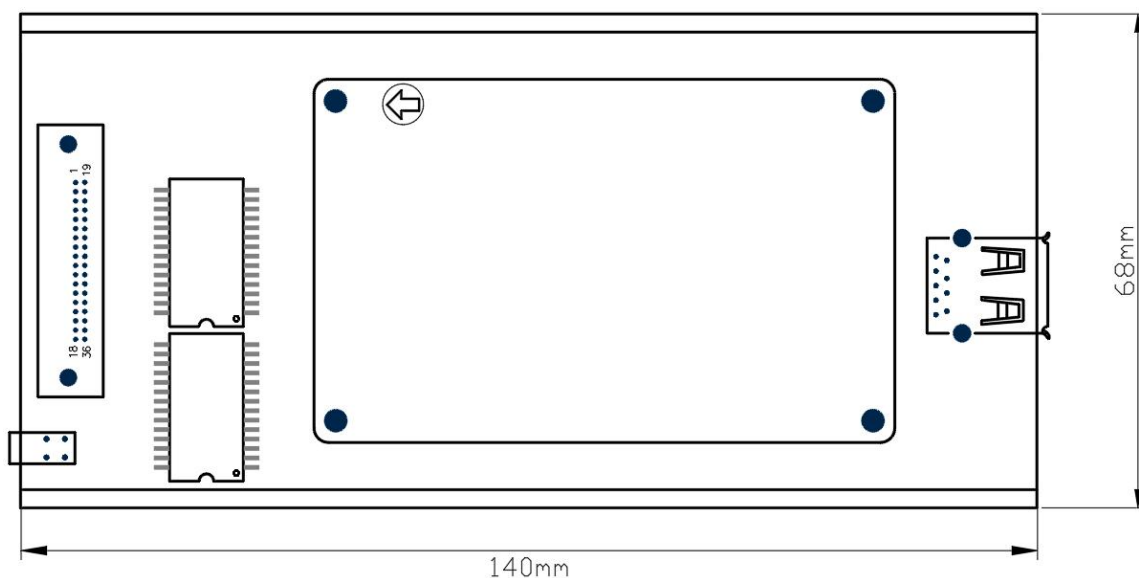
图 3 结构尺寸图
