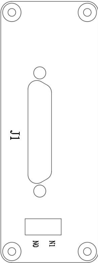
图 4 模块面板图
