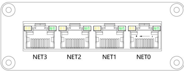
图 4 模块面板图
