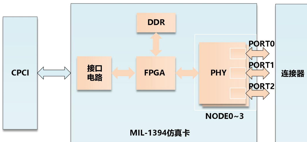
图 2 原理框图
