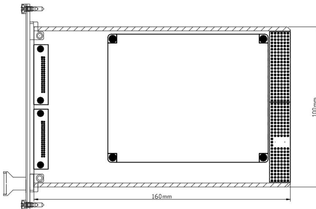
图 3 结构尺寸图
