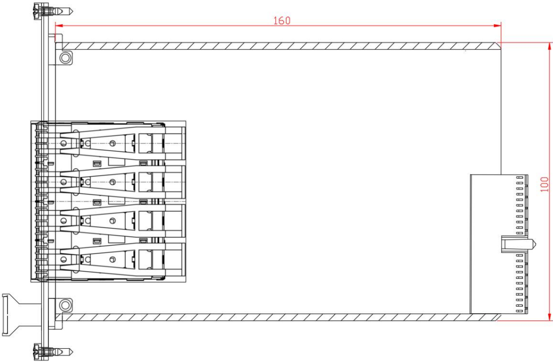
图 3 结构尺寸图
