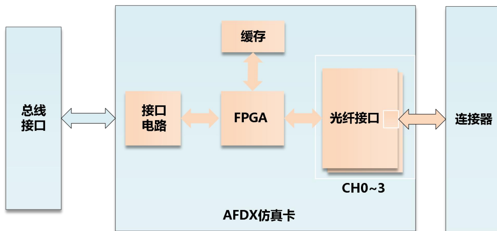
图 2 原理框图
