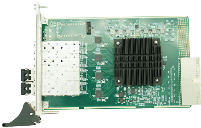
图 1 仿真板卡外观图
