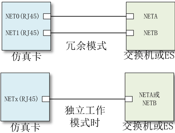
图 5 硬件接口连接示意图
