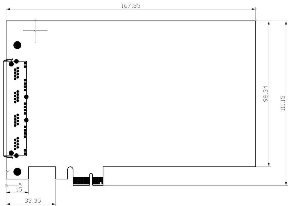
图 3 结构尺寸图
