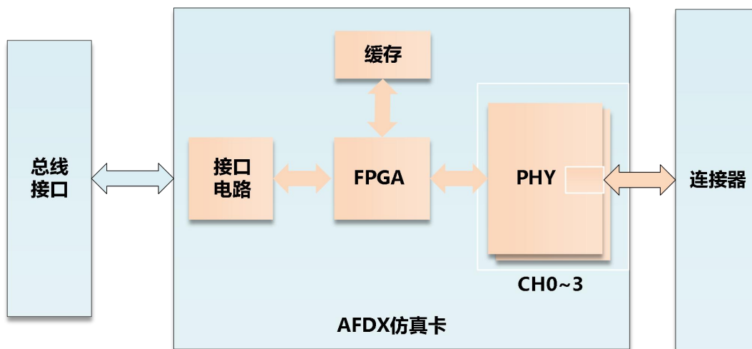
图 2 原理框图
