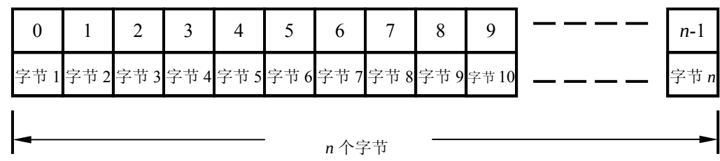
图 1-2.6.1.1 固定长度 Opaque 数据结构
