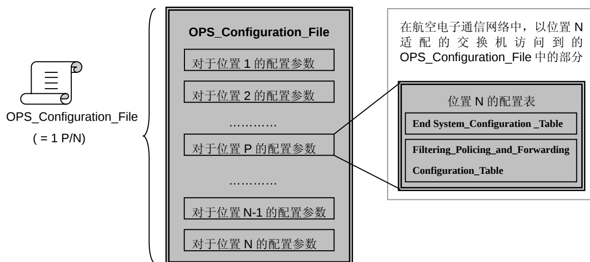
图 4-8 - OPS Configuration File 概况
