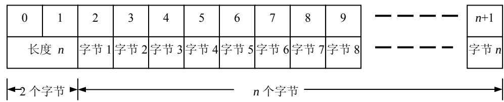
图 1-2.5.1 字符串数据结构格式
