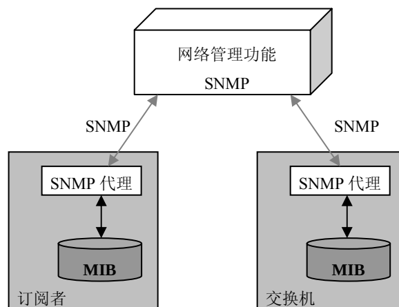
图 4-5 – 航空电子数据通信网络监视概况
