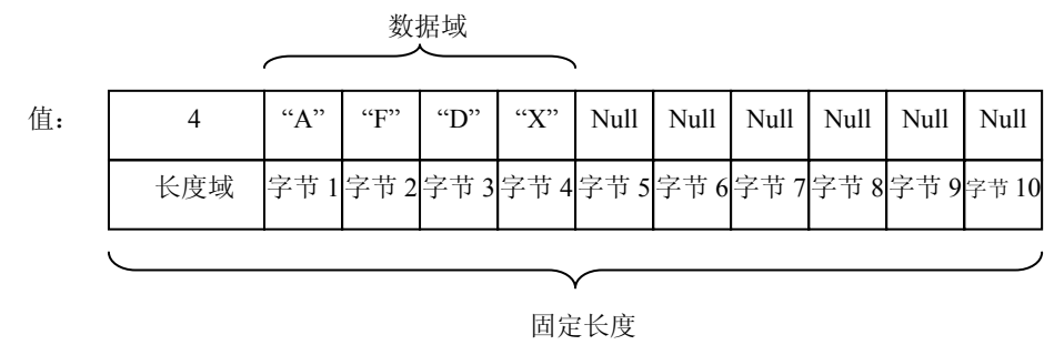
图 1-2.5.2 字符串数据结构
