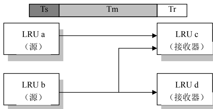
图 2-2 ARINC 429 总线
