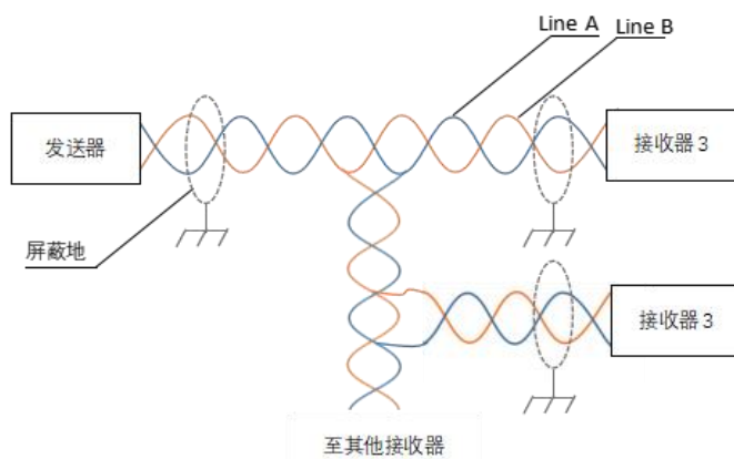
2 ARINC429 网络拓扑
